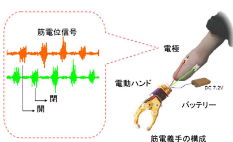
小児用筋電義手
